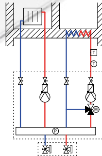
PHKR+MHKF Pumpen-Heizkreis für Radiatoren + Mischer- Heizkreis für Fußbo- den
